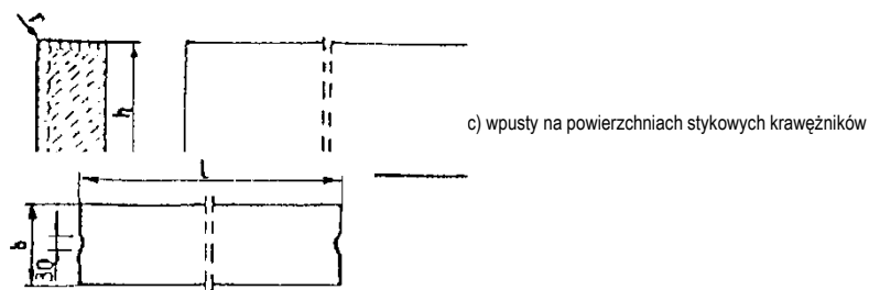
Rys. 1. Wymiarowanie krawężników
