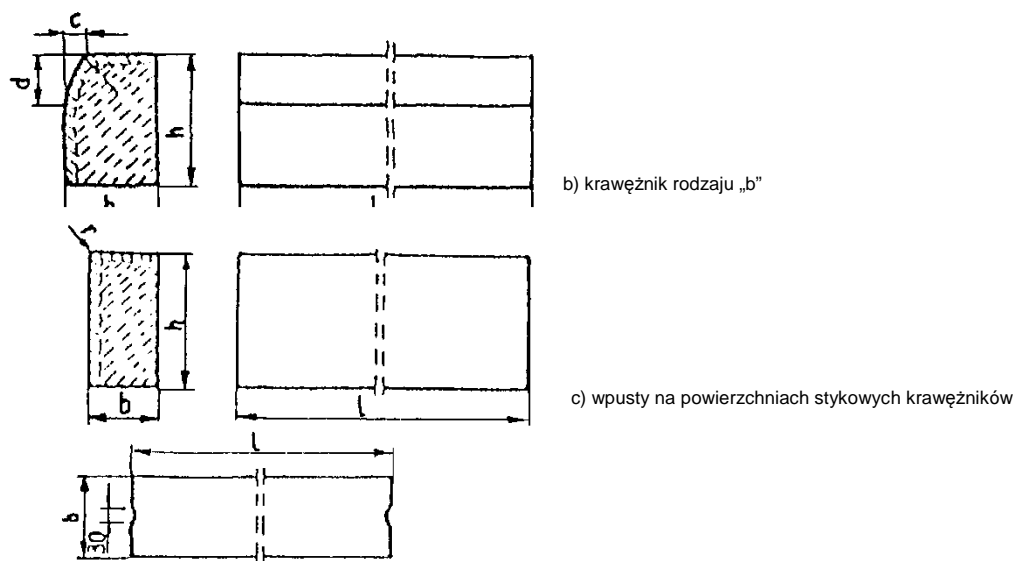
Rys. 1. Wymiarowanie krawężników
