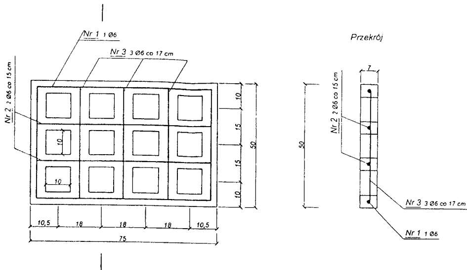
e) Płyta 0,75 x 0,50 x 0,07 m z otworami kwadratowymi
