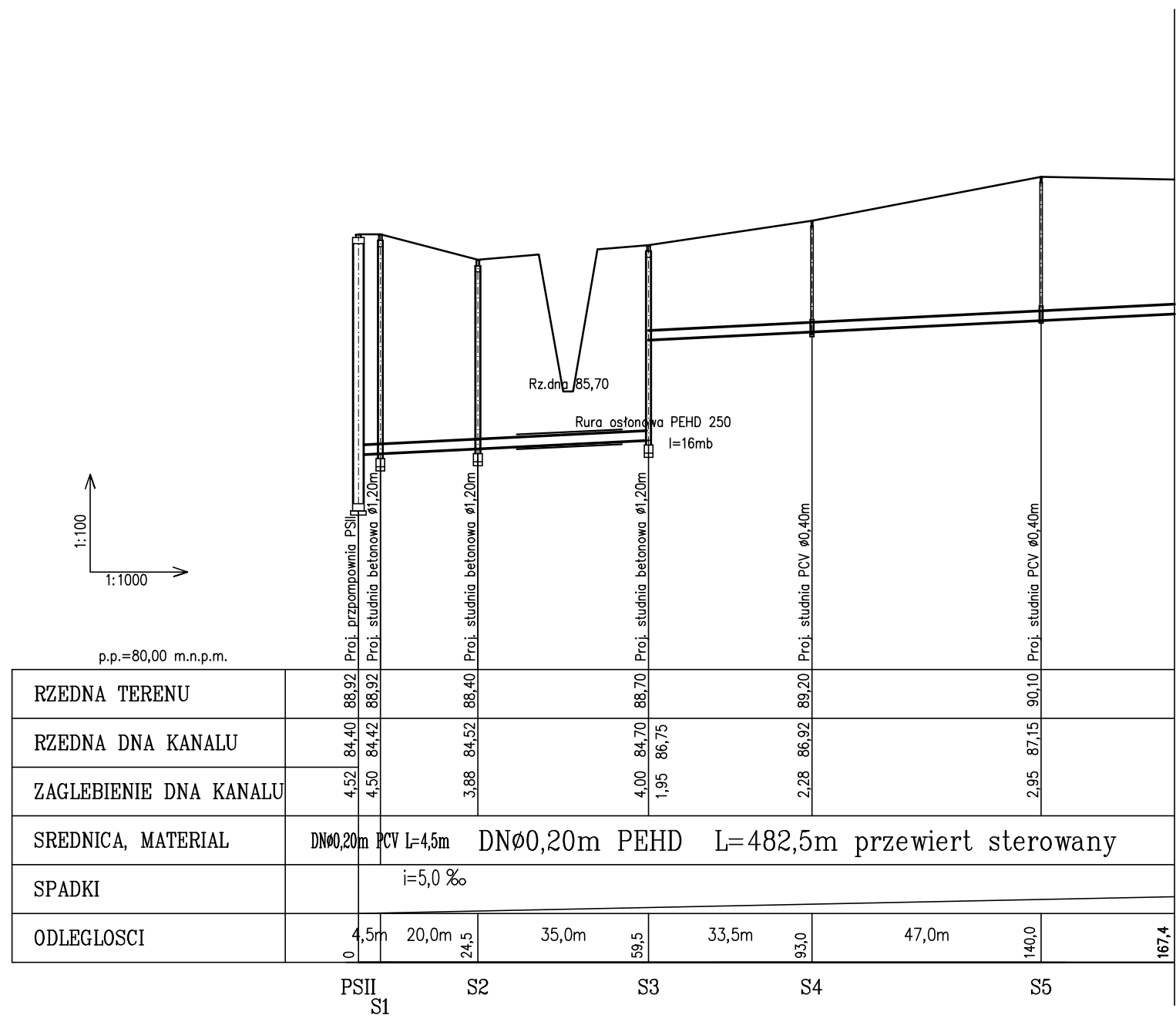
PROFIL PODŁUŻNY KANALU GRAWITACYJNEGO przejście pod rzeką Chełmiczką 1: \frac{100}{1000}
